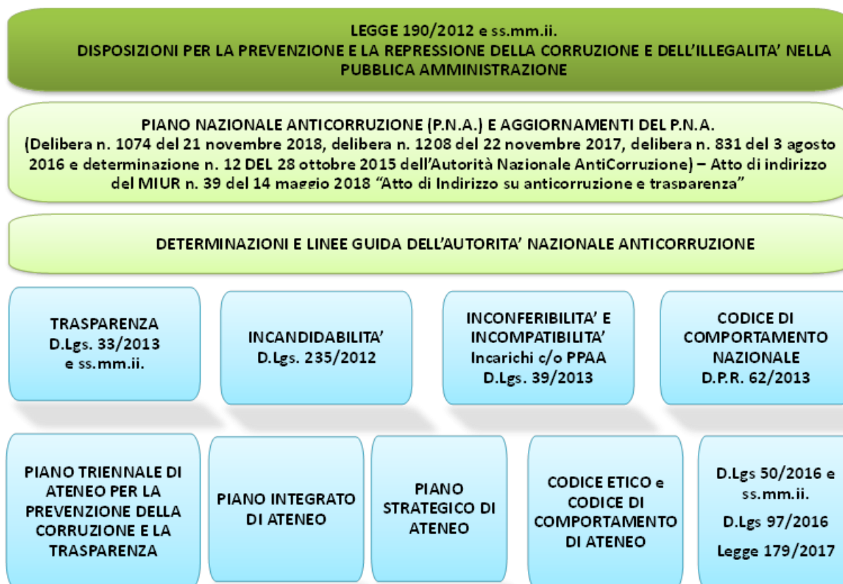
Figura 1: Assetto normativo
